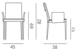
Bassa con braccioli GMVC
